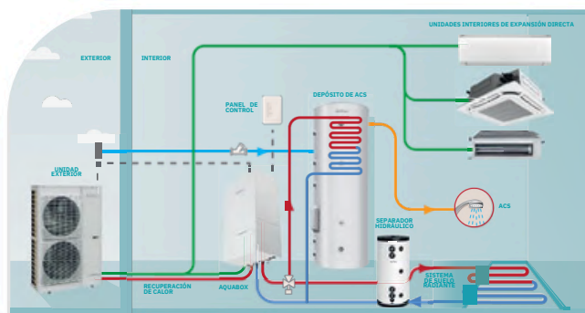
Aplicación mixta con Aquabox, depósito de ACS, sistema de suelo radiante y expansión directa
