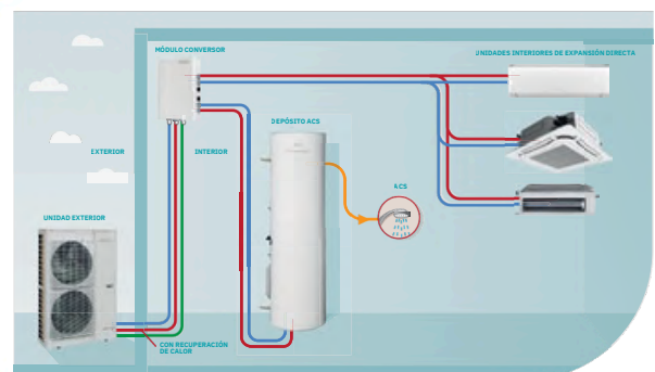
Aplicación mixta con generador de ACS y expansión directa
